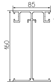
Guida portante con carter di chiusura
